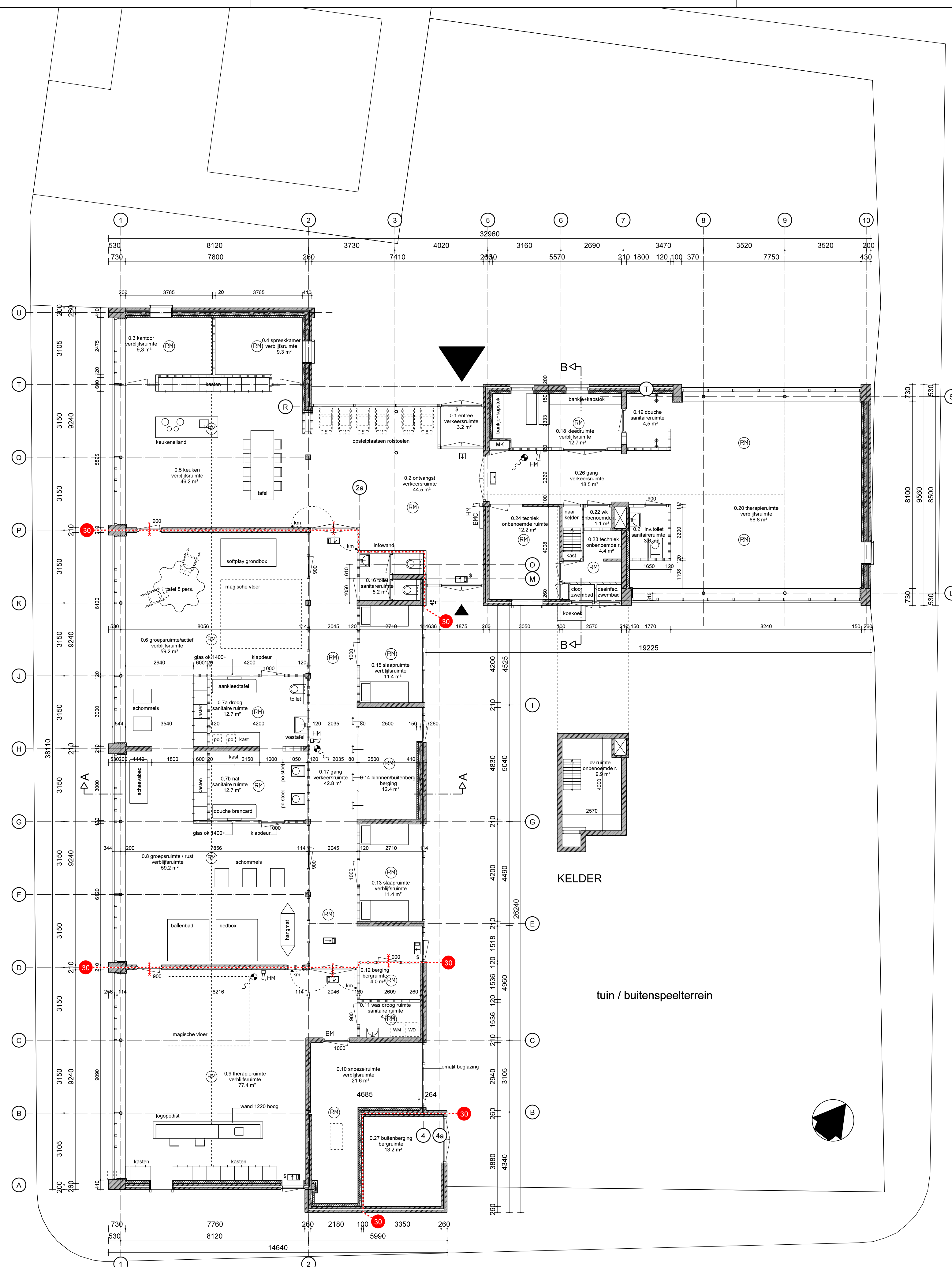
PLATTEGROND - BEGANE GROND nieuwe toestand
